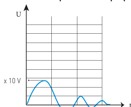
Четвертьволновой разрядник
